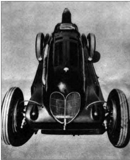
L'Alfa Romeo Bimotore è la prima vettura da corsa prodotta a Modena presso la Scuderia Ferrari nel 1935. Si trattava di una Tipo B-P3 modificata per alloggiare il secondo motore dietro il pilota. I serbatoi del carburante vennero sistemati in basso sulle fiancate.
