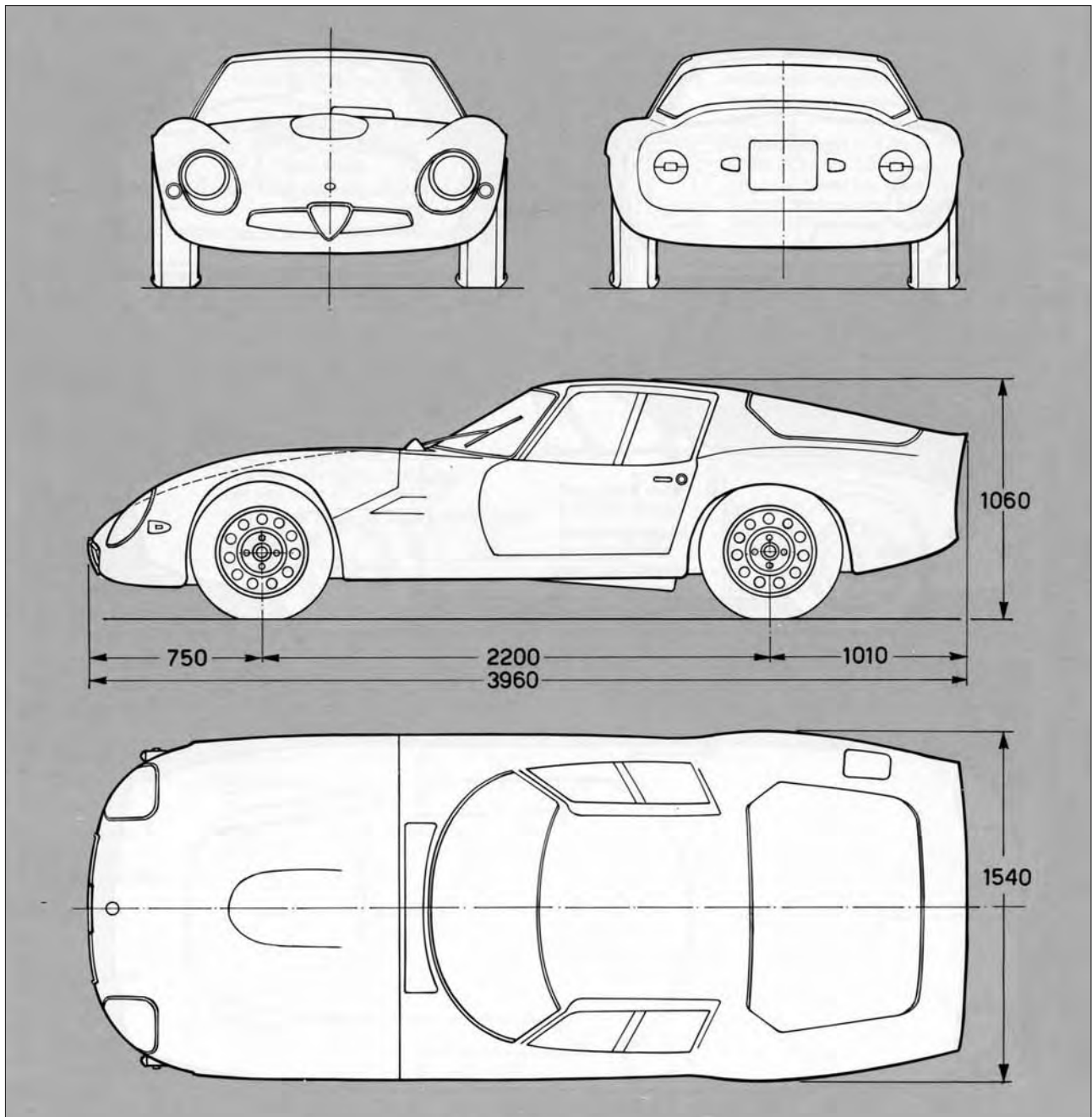
Le quattro viste quotate della TZ2 permettono di apprezzare le proporzioni, l'altezza di poco superiore a un metro, gli sbalzi contenuti sia anteriormente sia posteriormente, la coda Kamm.
