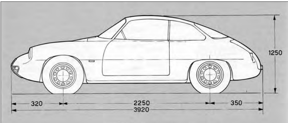
Il profilo della Giulietta SZ "coda tonda" prodotta dal 1960 al 1963 in 170 esemplari. Il motore 1290 cc erogava una potenza massima di 100 CV a 6.500 giri/min. Con la carrozzeria in alluminio il peso a vuoto era di 770 kg
