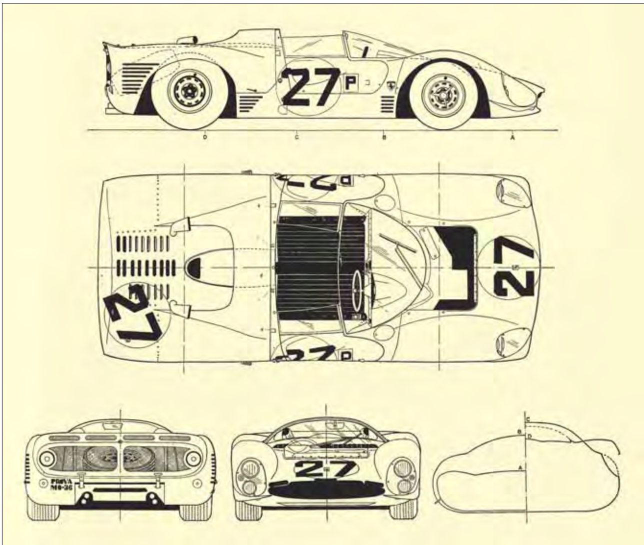
Il disegno della Ferrari 330 P3 in versione spider, utilizzata in parecchie corse nel 1966, tra le quali la 1000 Km del Nürburgring e la Targa Florio. Il risparmio di qualche kg nel peso non compensava il peggioramento della finezza aerodinamica rispetto alla versione berlina.
