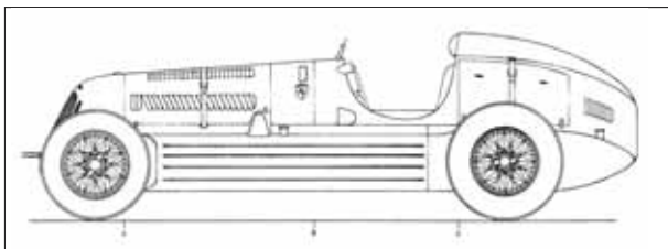
Profilo dell'Alfa Romeo Bimotore. Impossibile da guidare in circuito a causa dell'instabilità e dell'eccessivo consumo degli pneumatici, venne affidata al coraggio di Tazio Nuvolari che stabilì il primato internazionale Classe B sul km e miglio lanciati, 323, 125 km/h, autostrada Firenze-Mare.
