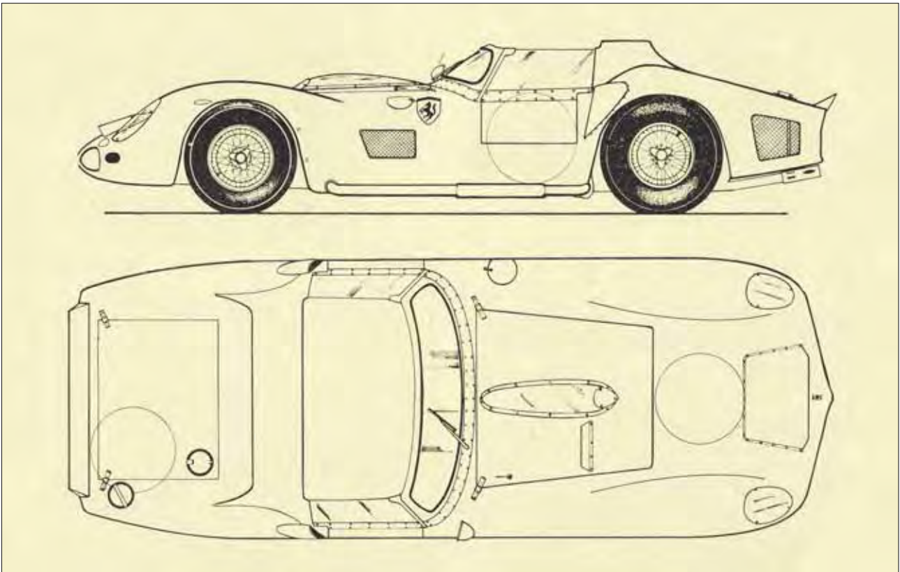
Profilo e pianta della Ferrari TRI-62, ultima vettura a motore anteriore che ha vinto a Le Mans, 1962. La guidavano Phil Hill-Olivier Gendebien. Il motore anteriore era il classico V12 Colombo da 4 litri. Lo studio aerodinamico appare particolarmente innovativo nella parte posteriore con la presenza del roll-bar carenato, la coda bassa, il grande spoiler. L'equilibrio con la parte anteriore era ottenuto con un cofano motore deportante.
